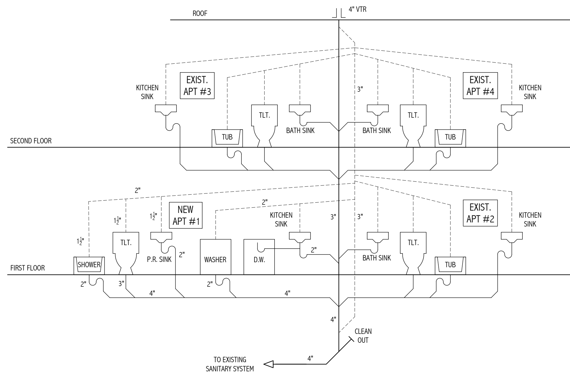
2 PLUMBING RISER DIAGRAM A-1 N.T.S.
