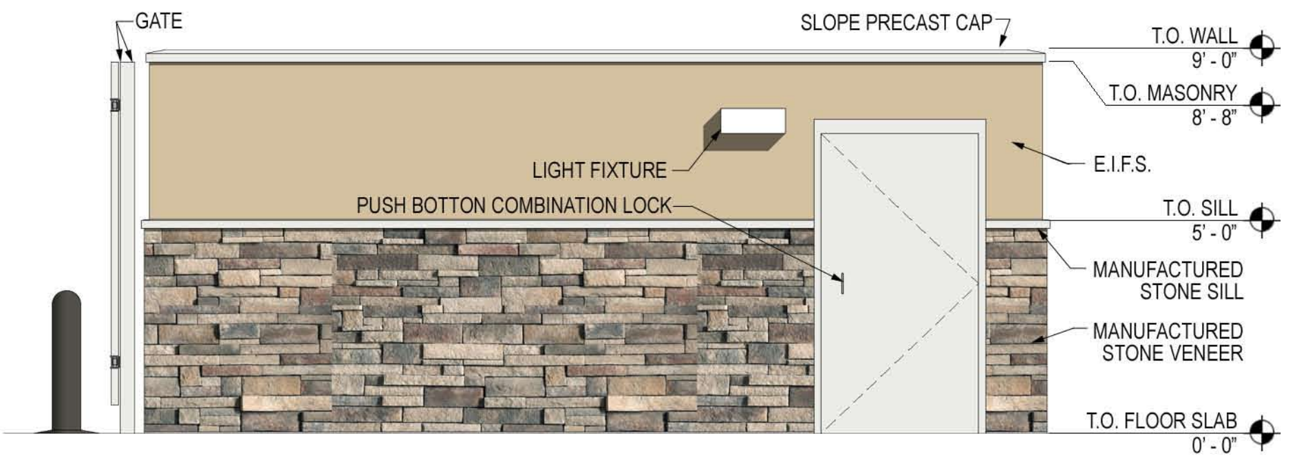
RIGHT ELEVATION
